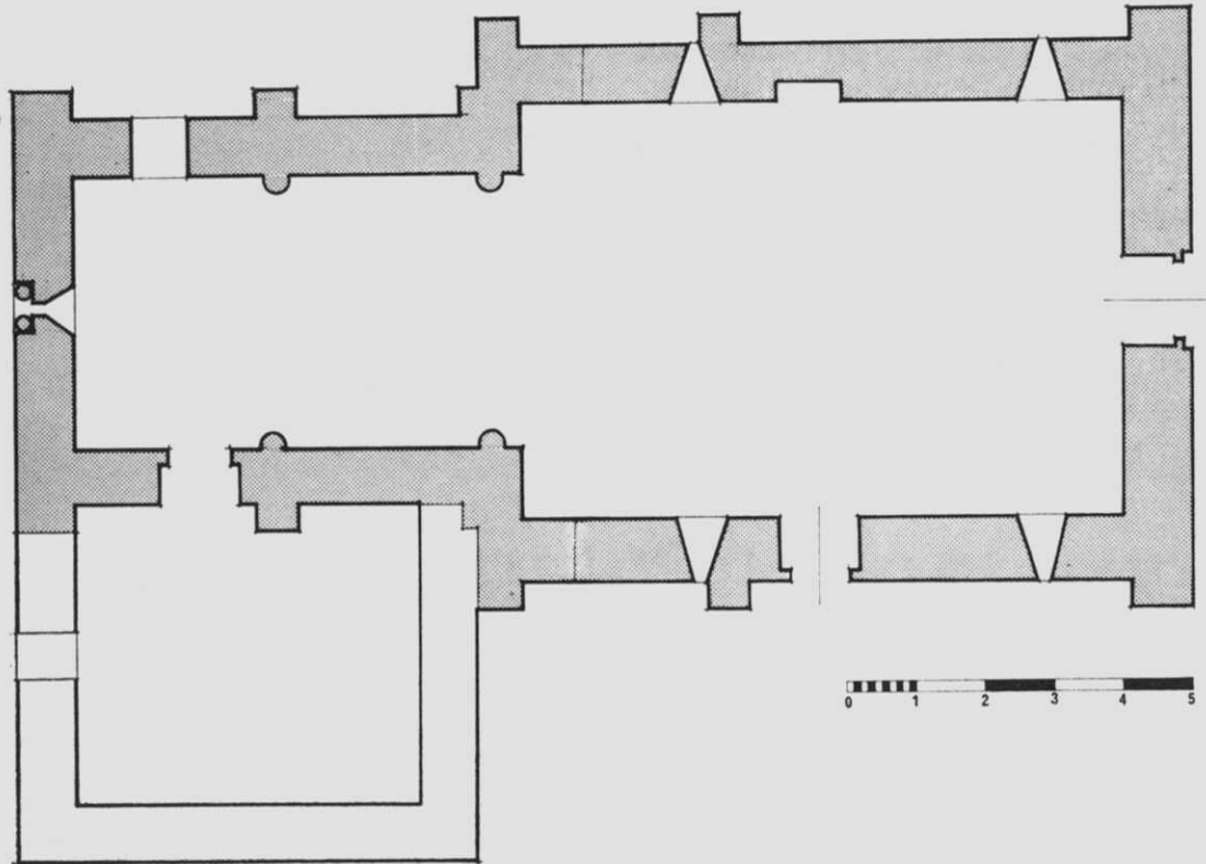
Eirexa de San Pedro de Oza dos Ríos.- Alzado lateral e planta. Por X. Ramón de Soraluce.
