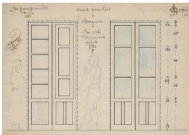
Arriba, deseño de «vidrieras de la fachada frontal» de casas xemelgas de Rois (Bergondo). 1925. AMB, c-7742 (procede da casa do autor).
