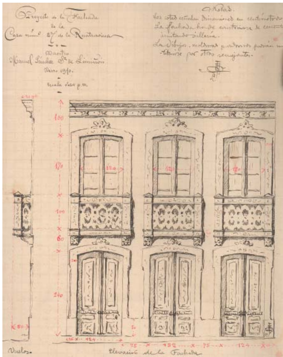
Proyecto de reconstrucción da casa número 27 da Rúa Travesa propiedade de D. Antonio López Dans. 1910. AMB, c-604.
