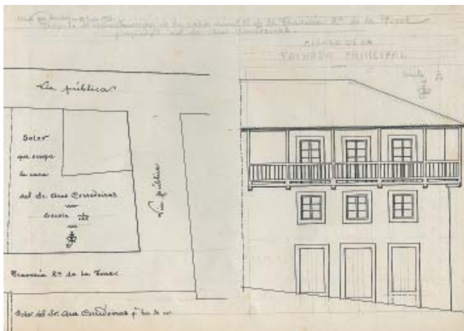
Borrador de proxecto de reconstrucción da casa número 11 da 2ª Travesía da Torre. AMB, c-7742 (procede da casa do autor).
