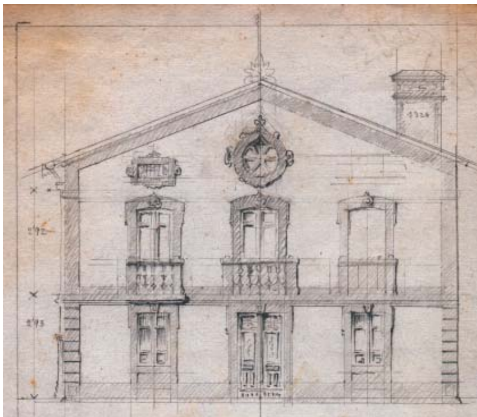
Borradores de fachadas, procedentes da casa do autor. AMB, c-7742.
