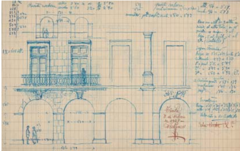
Borrador de proxecto de casa nos soportais do Campo. 1927. AMB, c-7742 (procedente da casa do autor).
