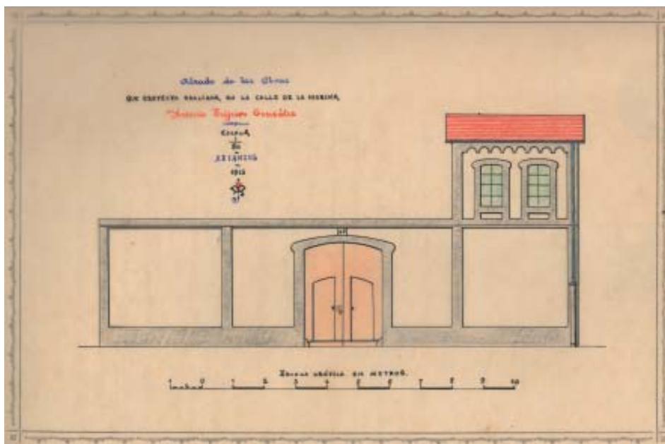
Proxecto instruído a instancia de D. Antonio Teijeiro González, solicitando permiso para reconstruir, formando unha soa finca, as casas números 24, 26 e 28 da rúa da Marina. Ano 1913. AMB, c-605.
