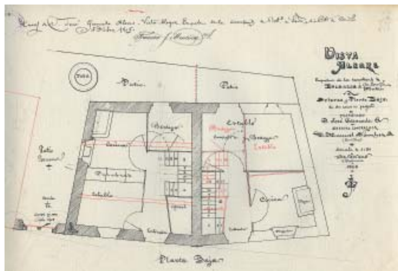
Borrador de proxecto da casa de D. José Germade en Vista Alegre, Betanzos. 1905. AMB, c-4394 (procede da casa do autor).
