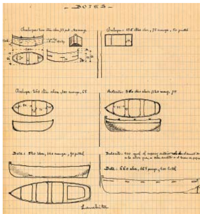
Borradores. Botes. Sen data. AMB, c-7742 (proceden da casa do autor).
